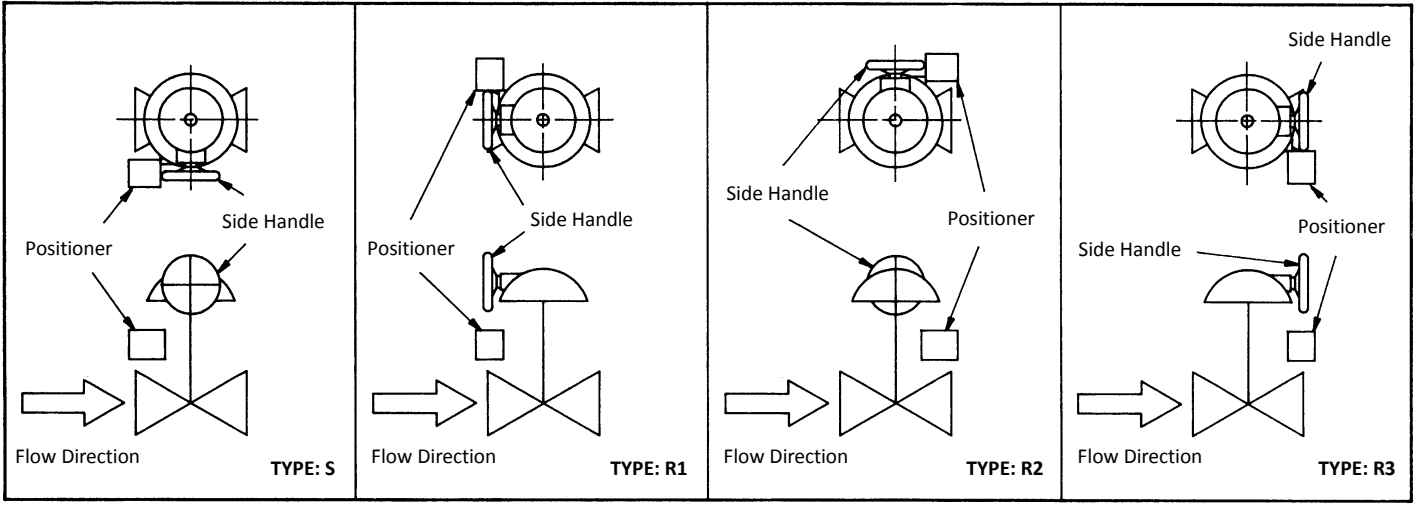
Fig. 6-2 ACTUATOR SIZE: 650
