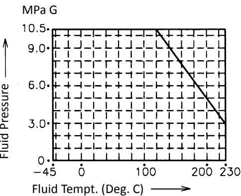
Fig. 2-1 R.TFE V-RING
