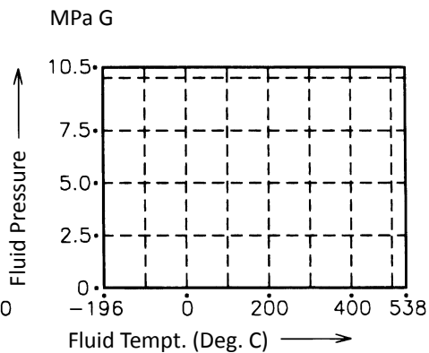
Fig. 2-3 GRAFOIL
