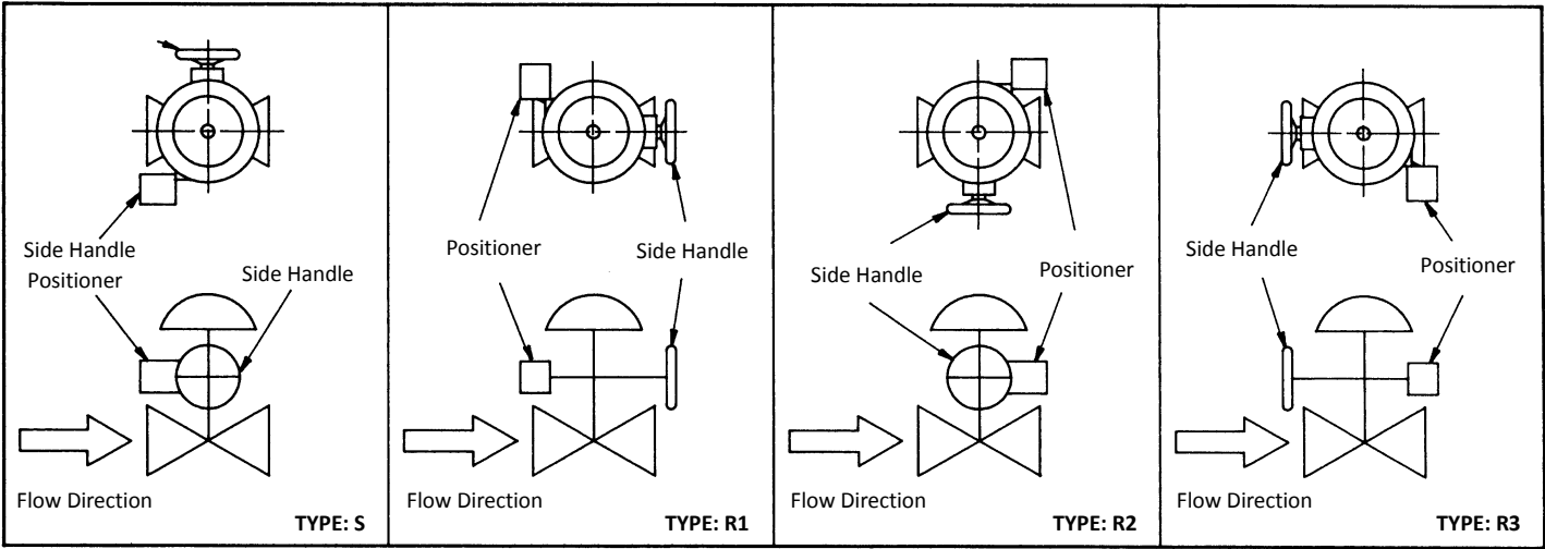
Fig. 6-1 ACTUATOR SIZE: 218~450
